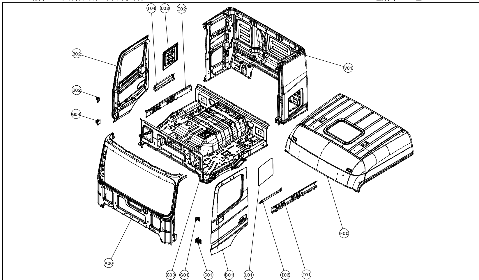
北奔 V3 车备件图册（白车身部分）
